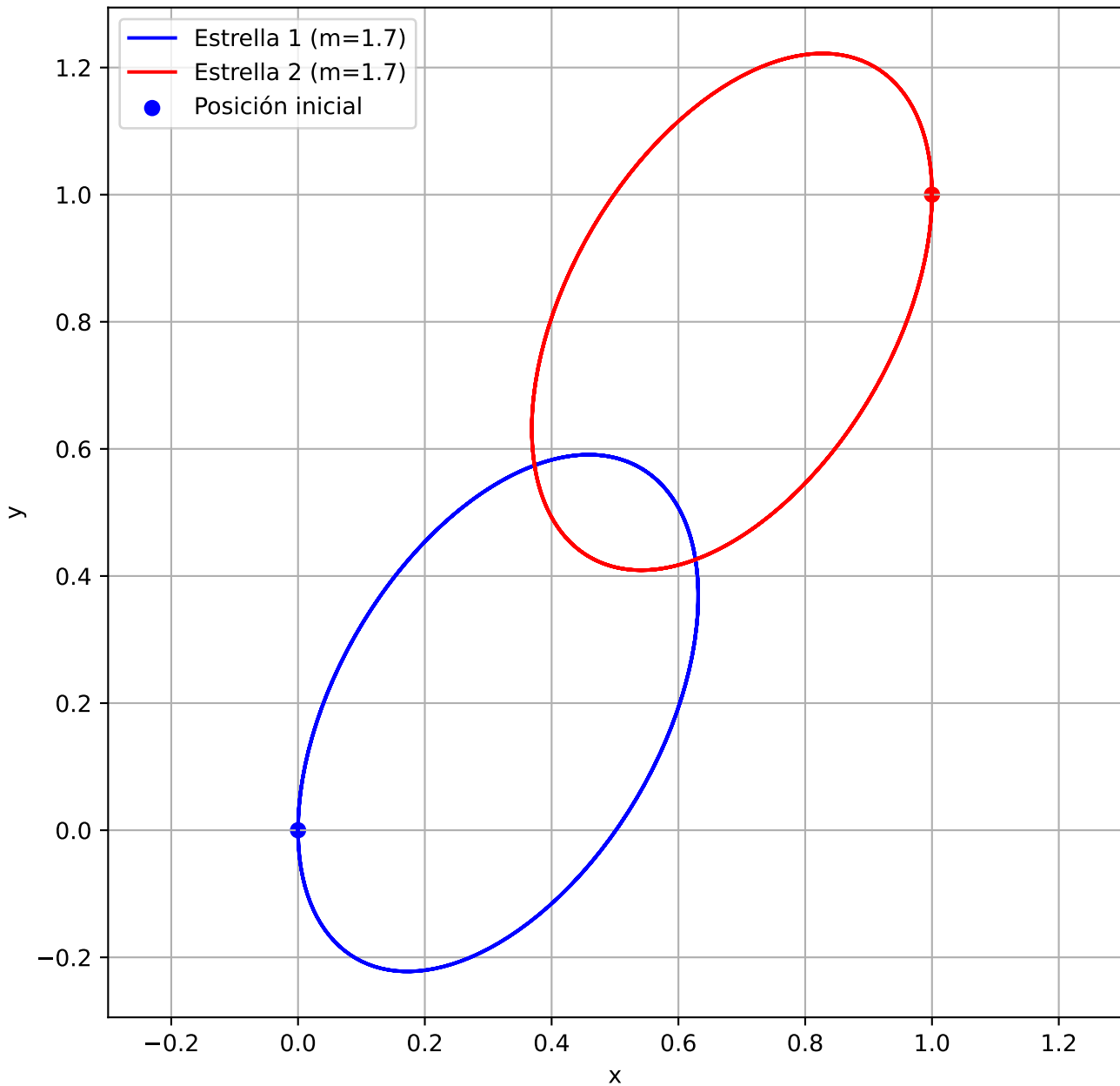
Órbita de un sistema binario con RK45
