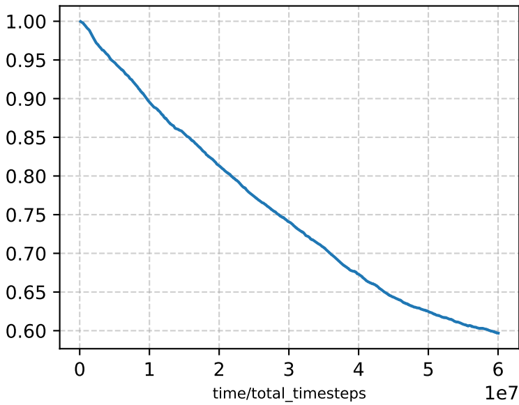
train/policy_gradient_loss
