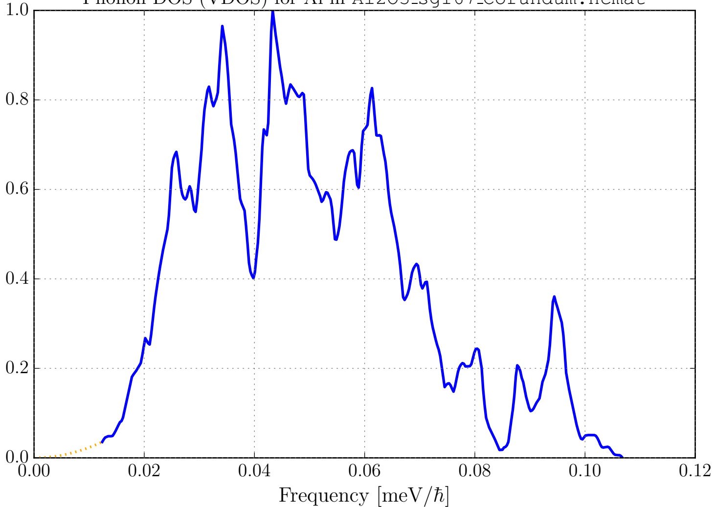
Phonon DOS (VDOS) for Al in Al 2 O 3 _sg167_Corundum.ncmat
