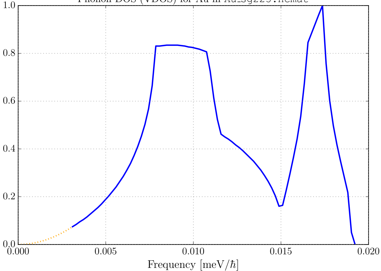
Phonon DOS (VDOS) for Au in Au_sg225.ncmat
