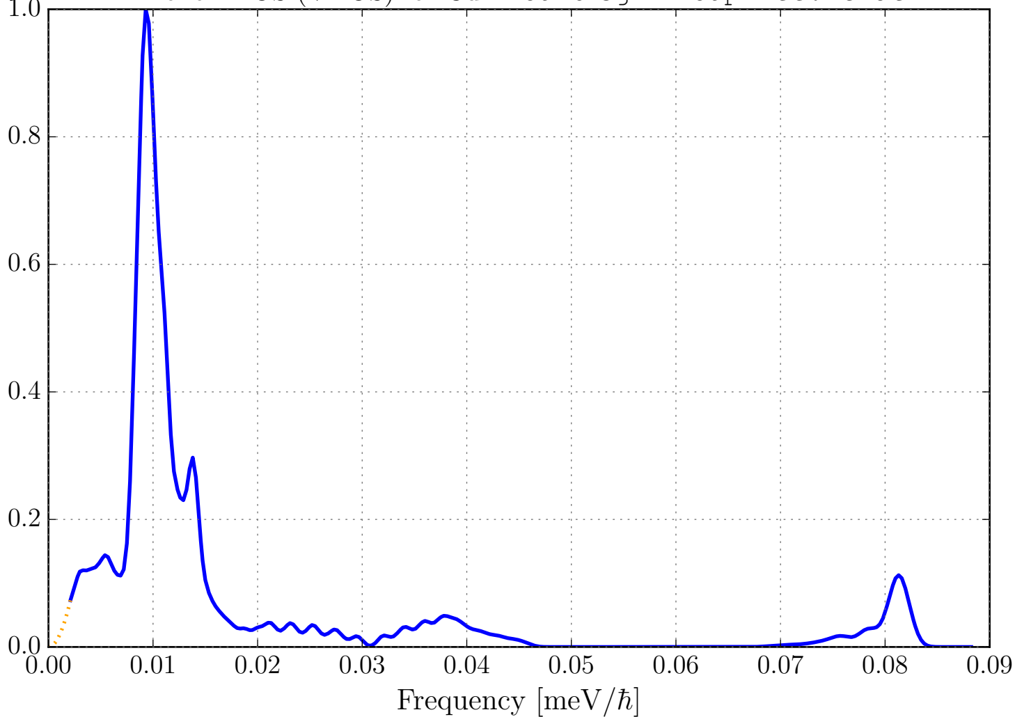
Phonon DOS (VDOS) for Cu in Cu 2 O_sg224_Cuprite.ncmat
