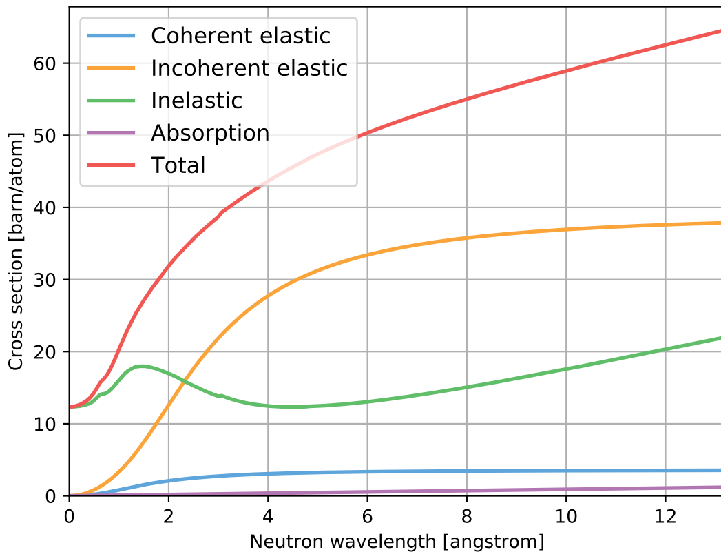
Epoxy_Araldite506_C18H20O3.ncmat
