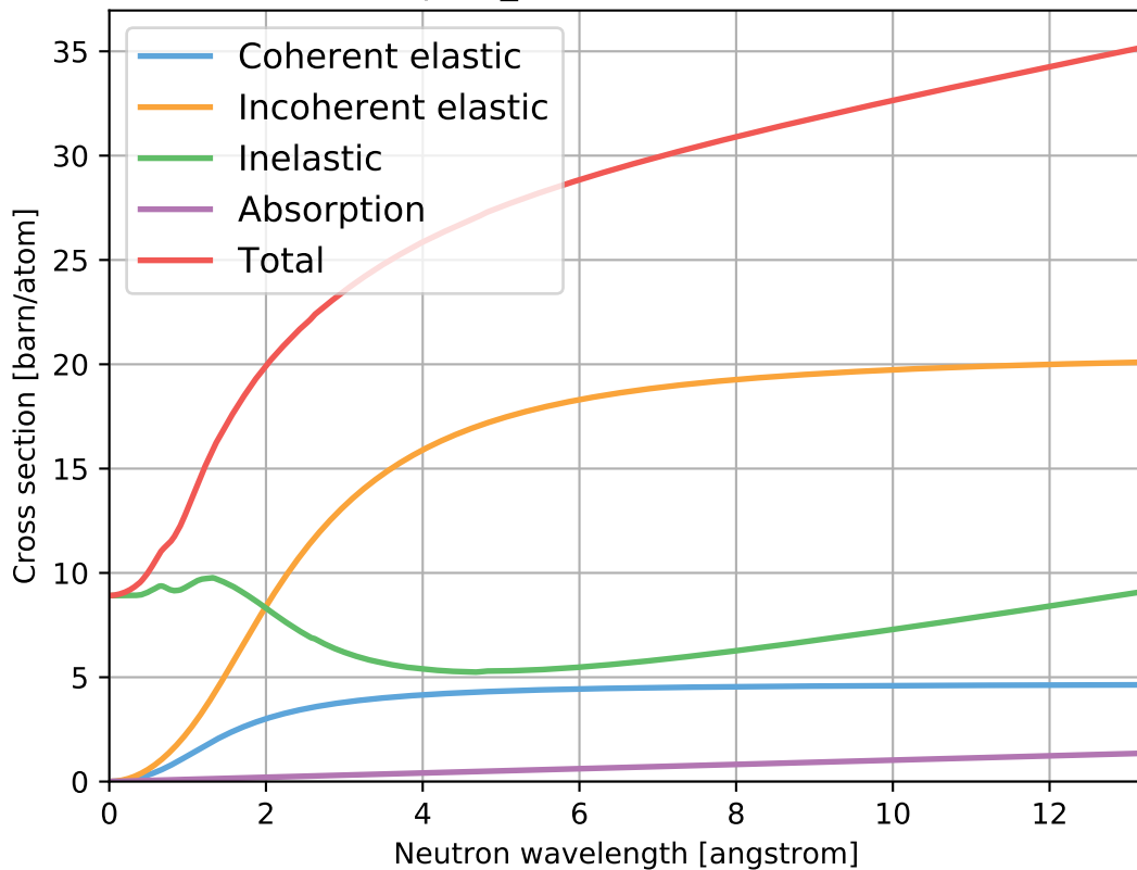
Kapton_C22H10N2O5.ncmat
