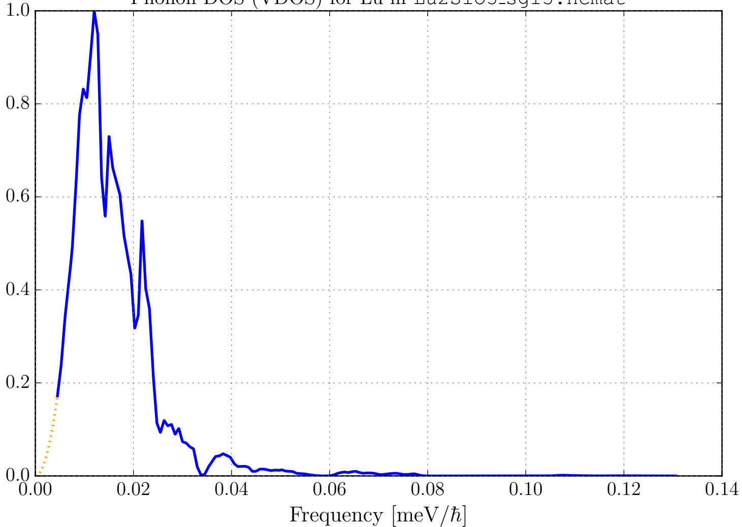
Phonon DOS (VDOS) for Lu in Lu 2 SiO 5 _sg15.ncmat
