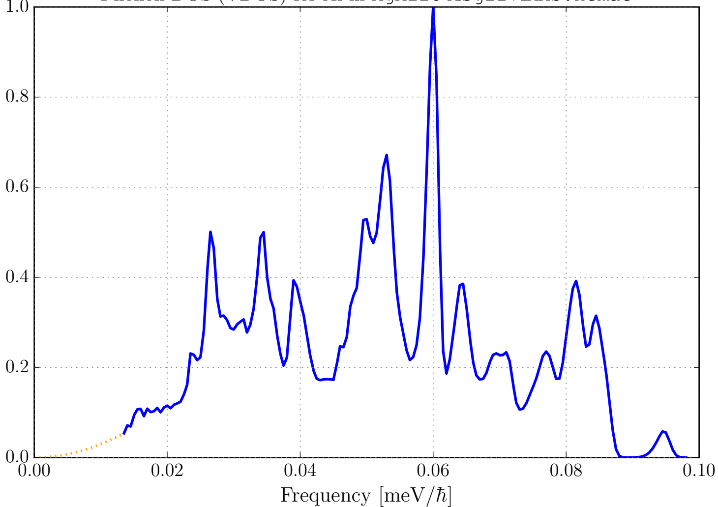
Phonon DOS (VDOS) for Al in MgAl 2 O 4 _sg227_MAS.ncmat
