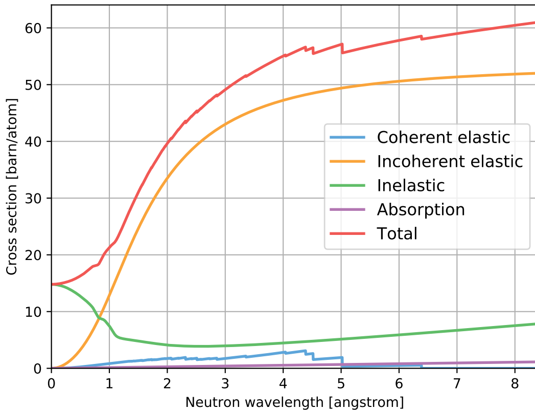
MgH2_sg136_MagnesiumHydride.ncmat
