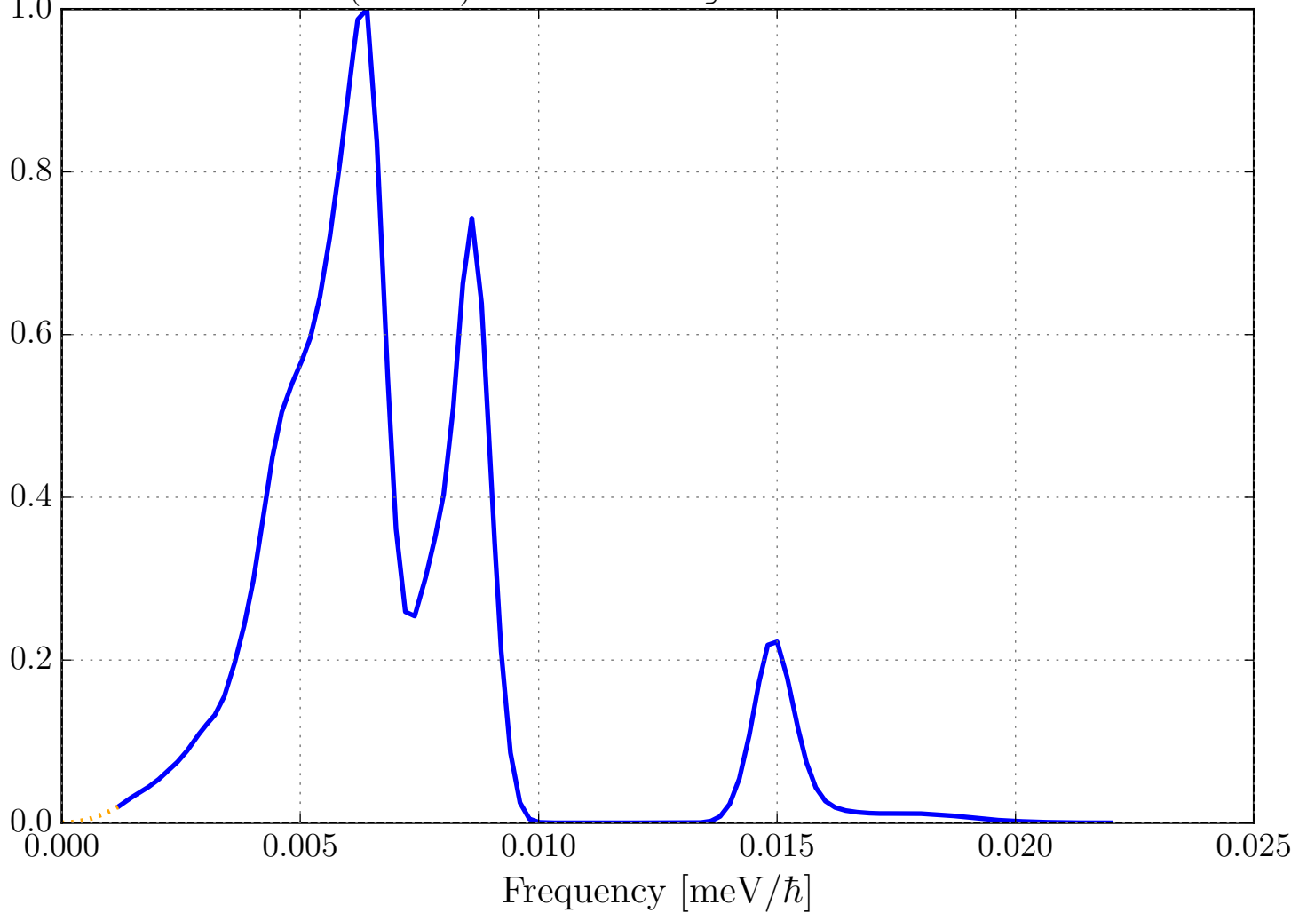
Phonon DOS (VDOS) for I in NaI_sg225_SodiumIodide.ncmat
