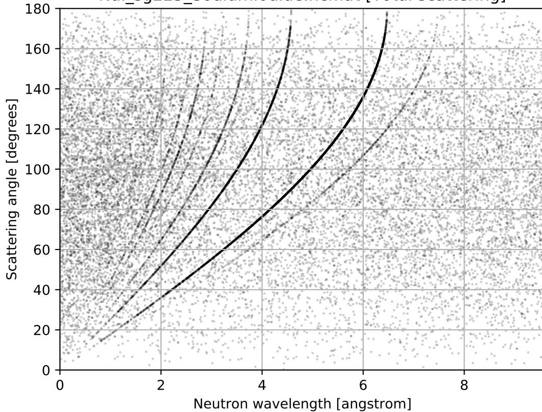
NaI_sg225_SodiumIodide.ncmat [Total scattering]
