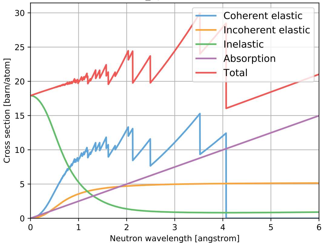
Ni_sg225.ncmat
