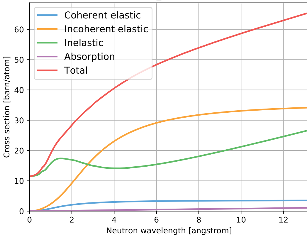
Polylactide_C3H4O2.ncmat
