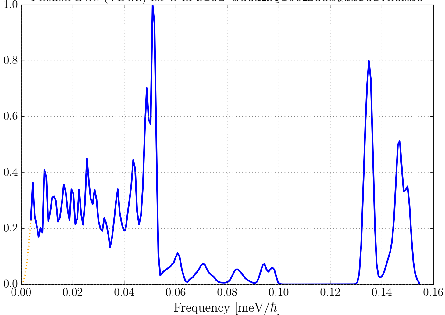
Phonon DOS (VDOS) for O in SiO2-beta_sg180_BetaQuartz.ncmat
