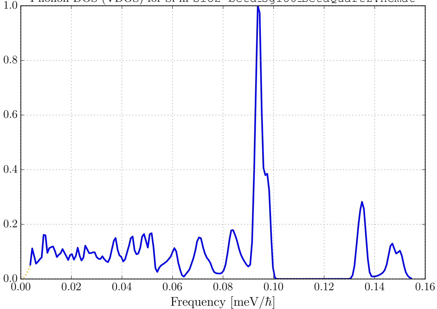
Phonon DOS (VDOS) for Si in SiO2-beta_sg180_BetaQuartz.ncmat
