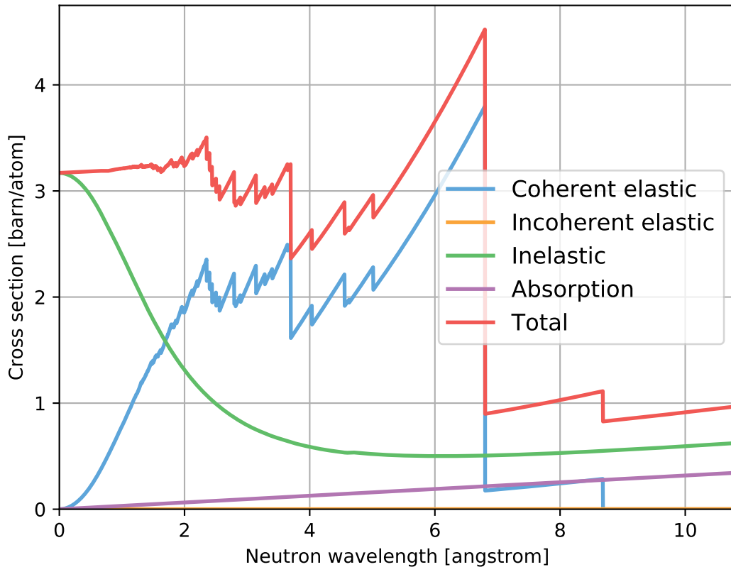
SiO2-beta_sg180_BetaQuartz.ncmat
