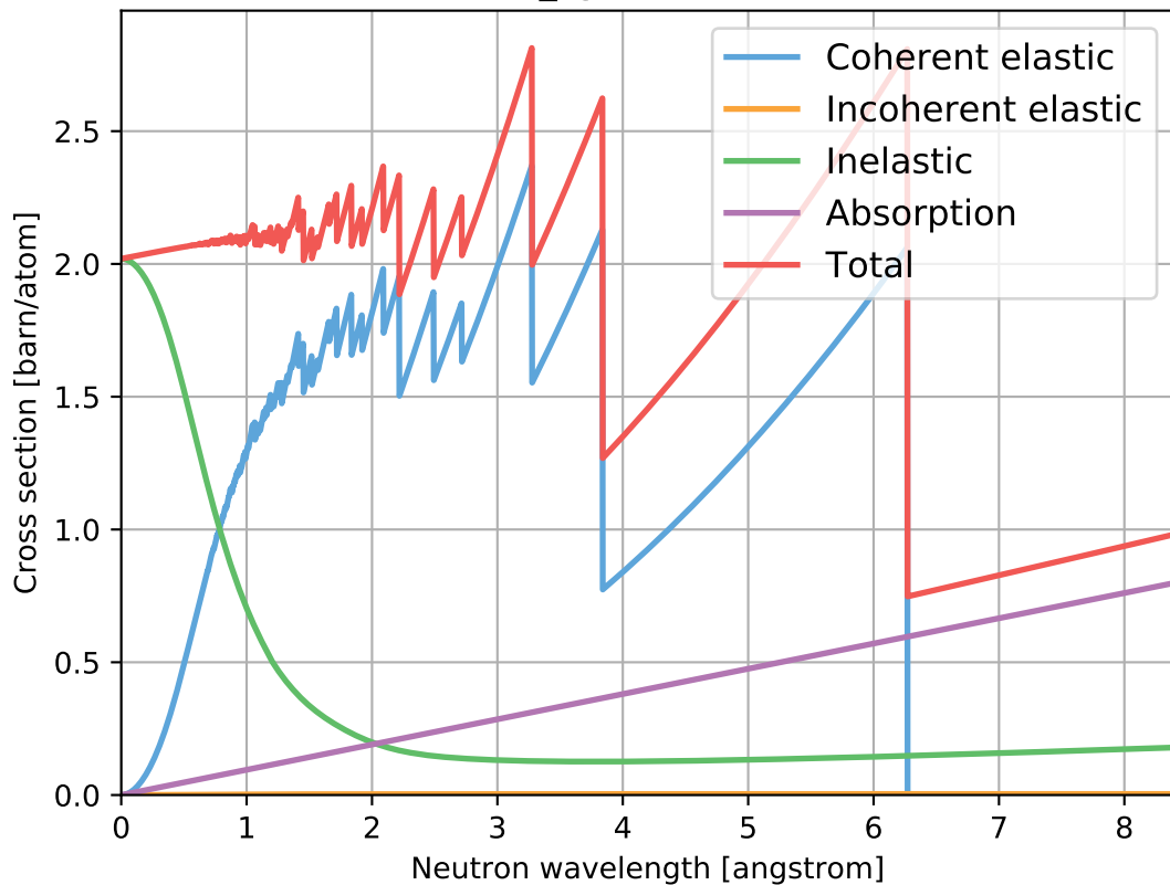
Si_sg227.ncmat
