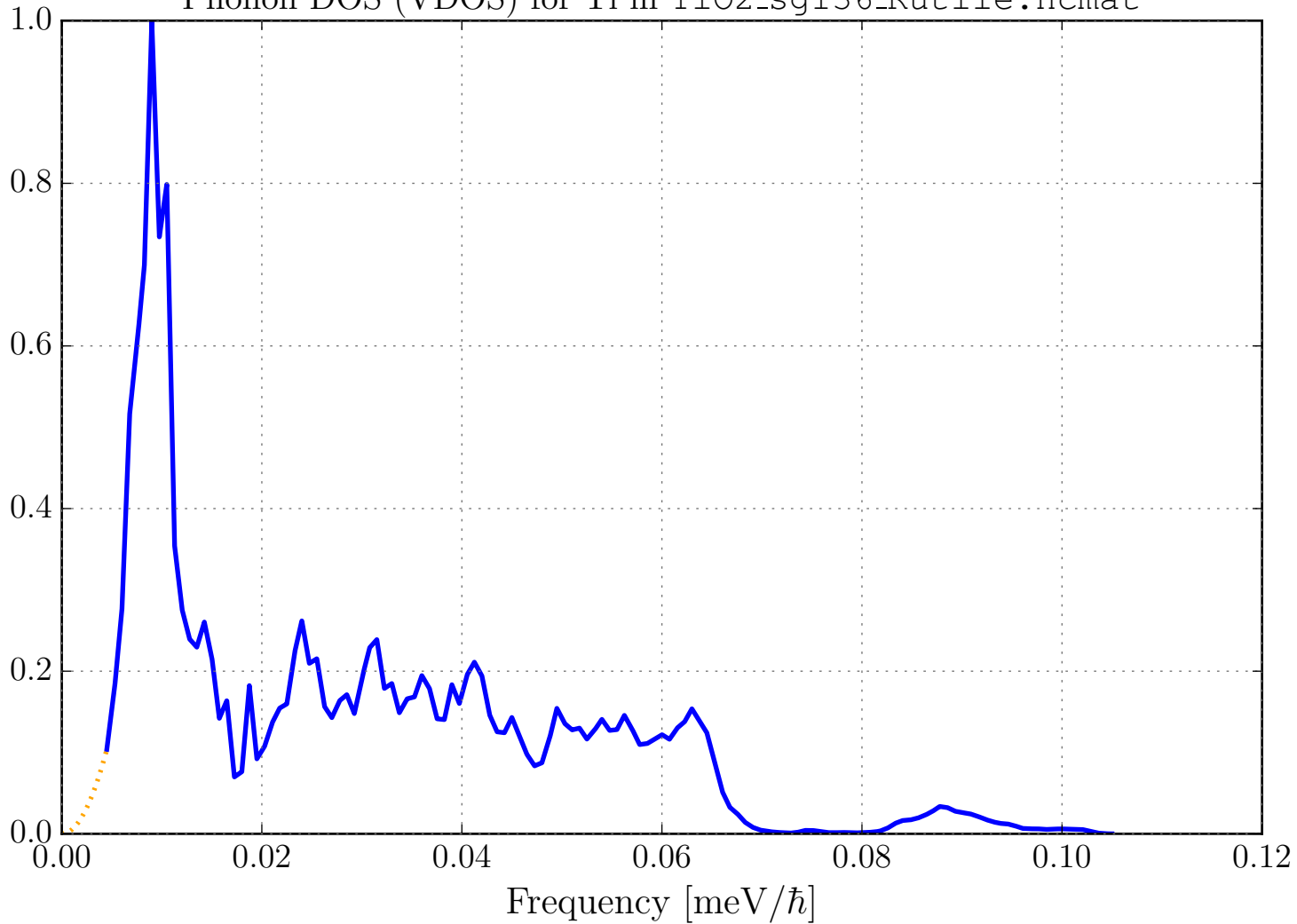
Phonon DOS (VDOS) for Ti in TiO2_sg136_Rutile.ncmat
