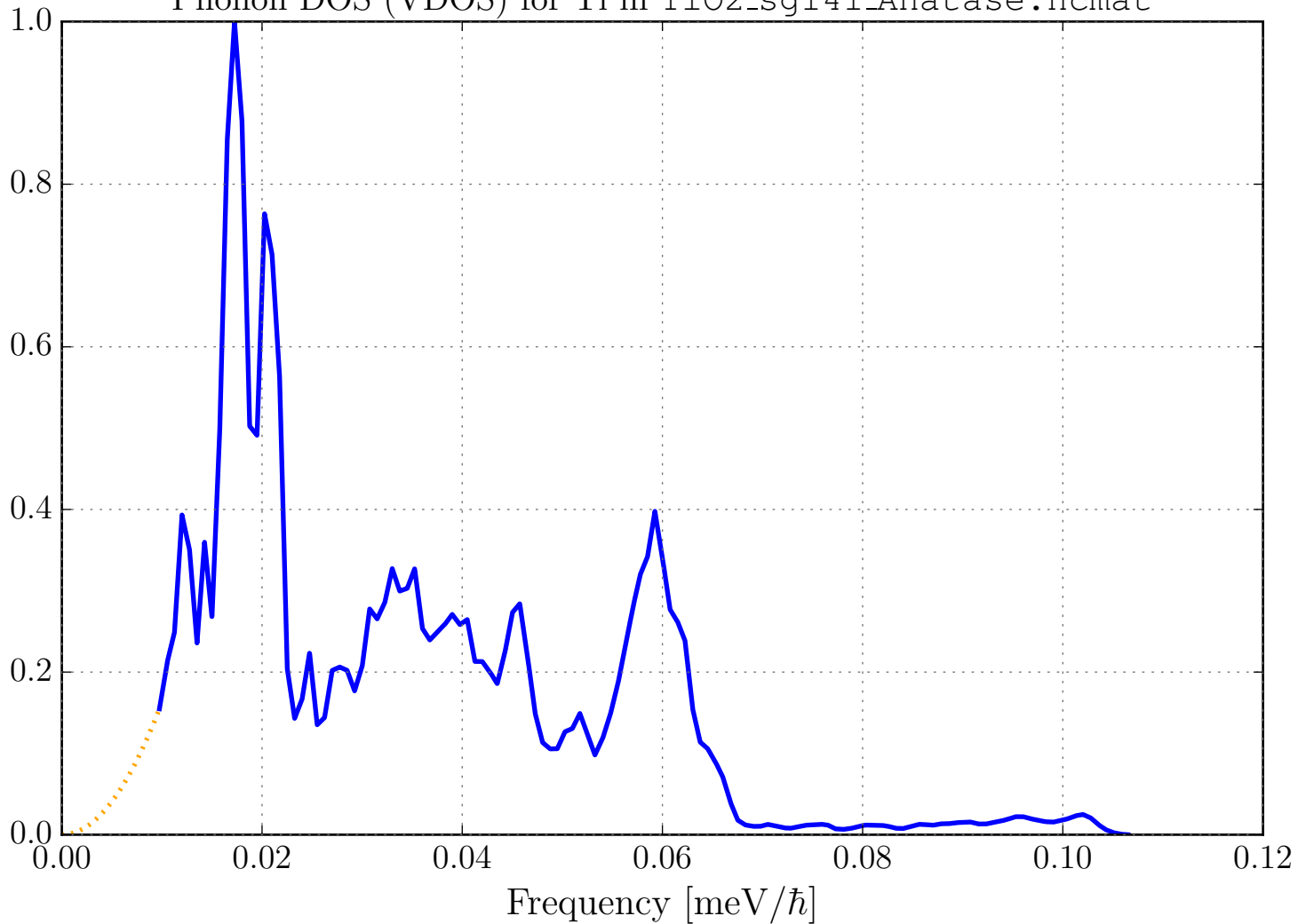
Phonon DOS (VDOS) for Ti in TiO2_sg141_Anatase.ncmat
