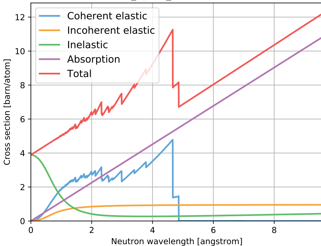
TiO2_sg141_Anatase.ncmat
