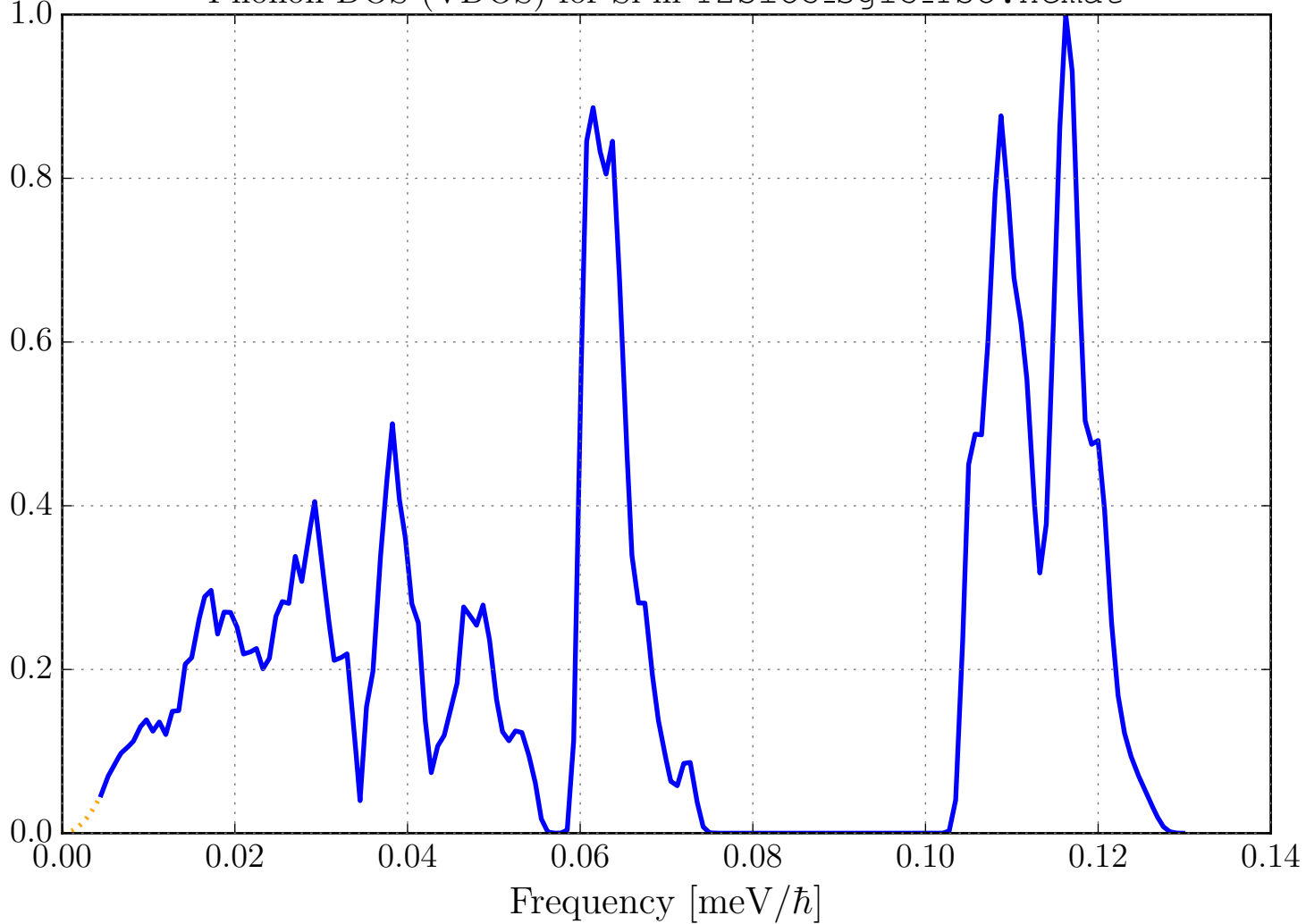
Phonon DOS (VDOS) for Si in Y2SiO5_sg15_YSO.ncmat
