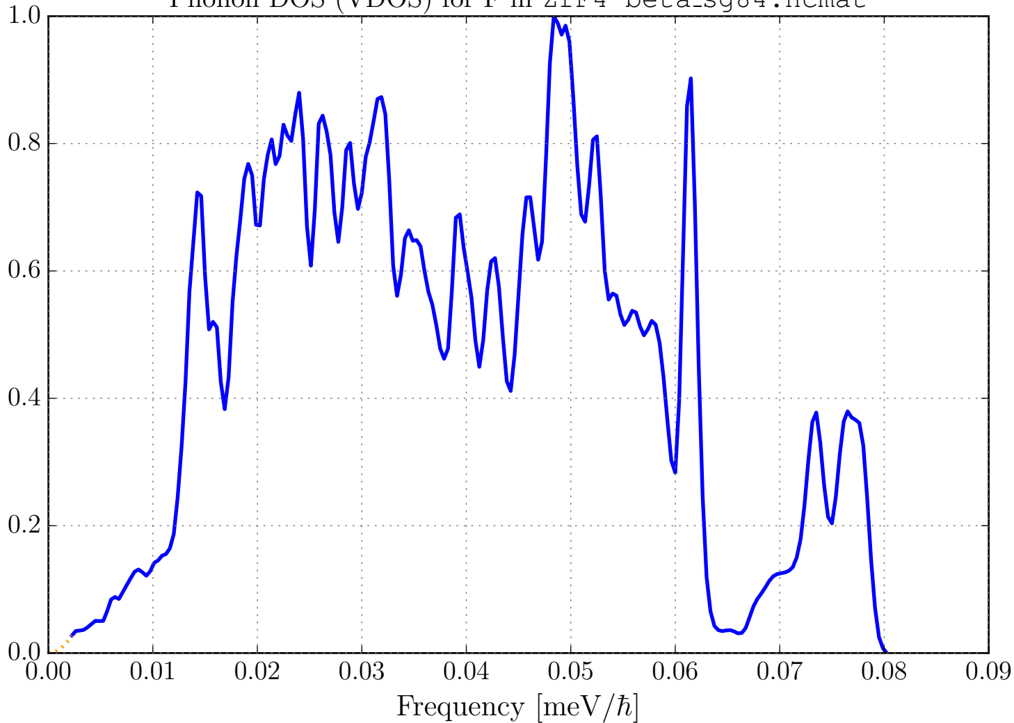
Phonon DOS (VDOS) for F in ZrF4-beta_sg84.ncmat
