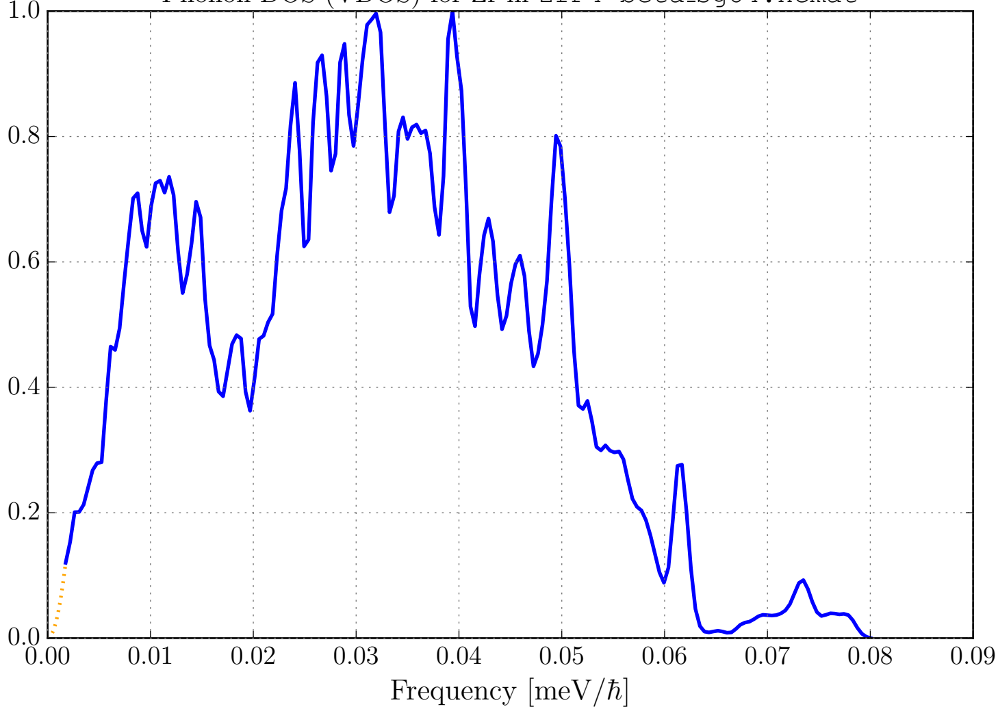
Phonon DOS (VDOS) for Zr in ZrF4-beta_sg84.ncmat
