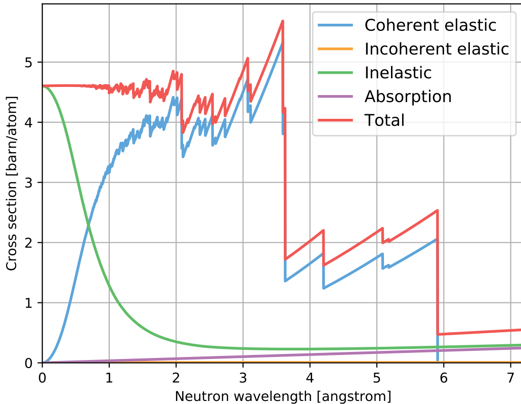
ZrO2_sg137_Zirconia.ncmat
