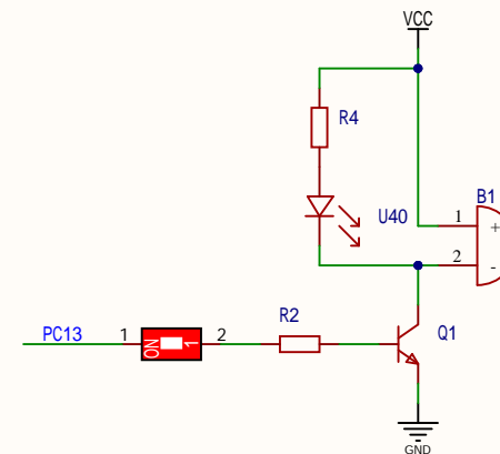
蜂鸣器
