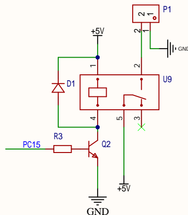
继电器
