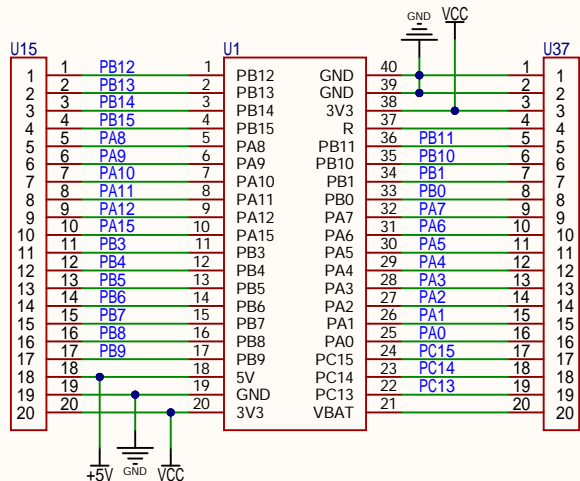
STM32F103C8T6最小系统板
