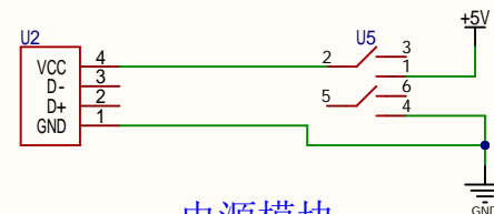
电源模块
