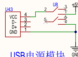
USB电源模块
