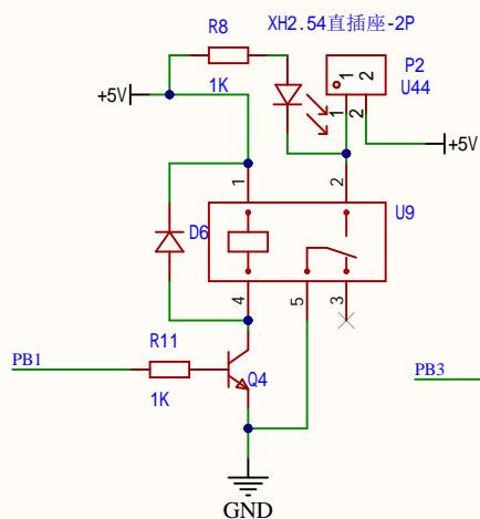
继电器（风扇）
