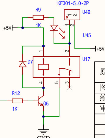
继电器（加热片）
