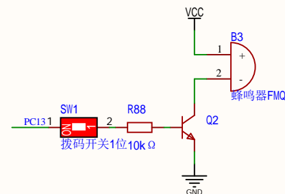
蜂鸣器报警
