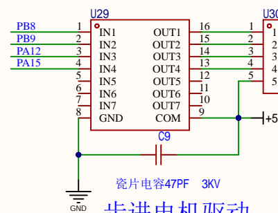
步进电机驱动
