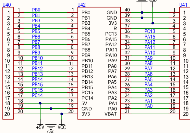
STM32F103C8T6最小系统板
