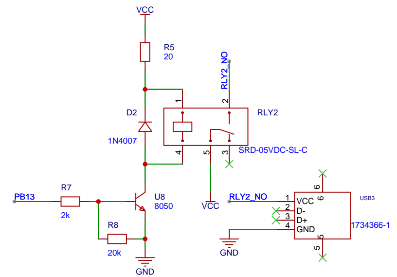
继电器2电路
