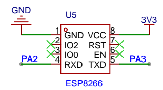
ESP8266模块
