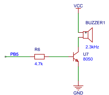
蜂鸣器电路
