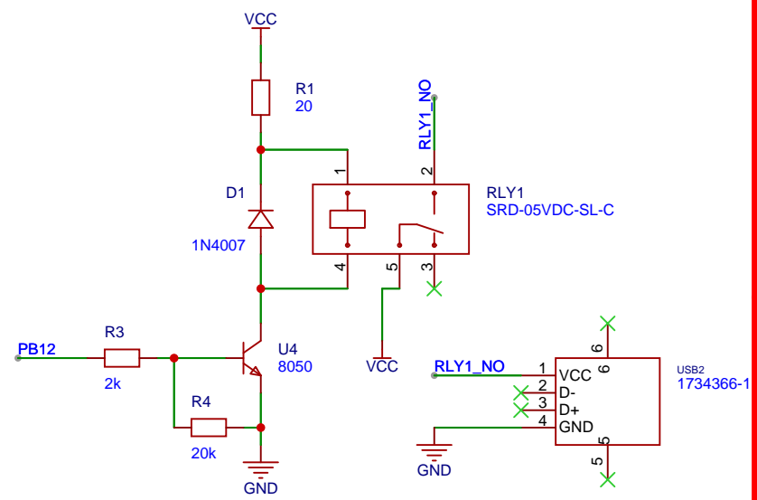
继电器1电路
