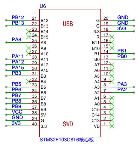
STM32核心板
