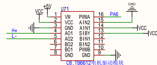
TB6612电机驱动
