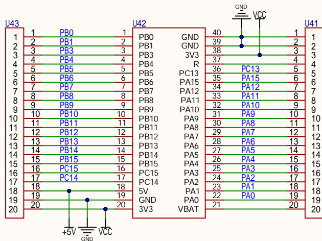
STM32F103C8T6最小系统板
