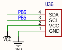
OLED屏幕
