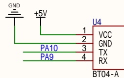
BT04-A蓝牙
