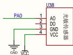
光敏传感器
