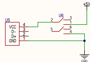
电源模块
