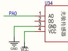
光敏电阻传感器
