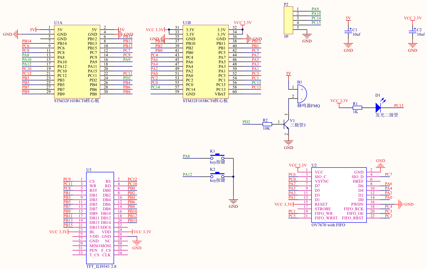
基于STM32F103车牌识别系统
