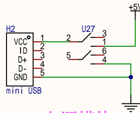
电源模块
