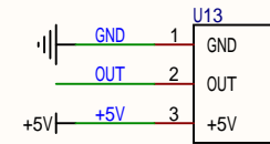
人体红外
