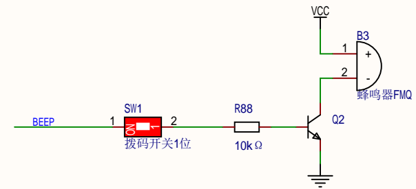
蜂鸣器
