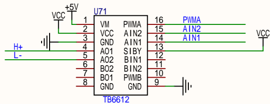
TB6612电机驱动
