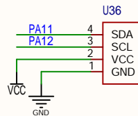
OLED屏幕
