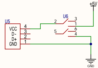
电源模块
