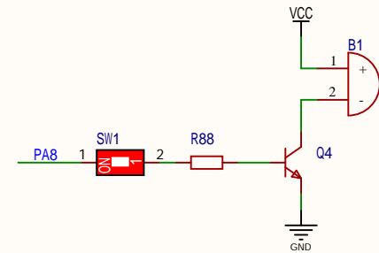
蜂鸣器
