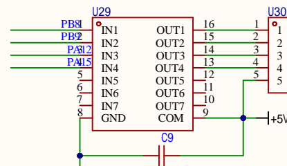
步进电机驱动
