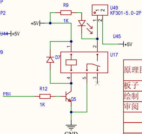
继电器 (加热片)
