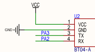
BT04-A蓝牙模块
