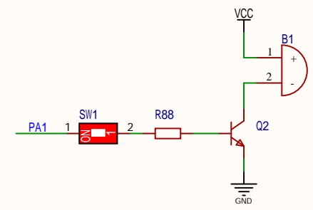
蜂鸣器
