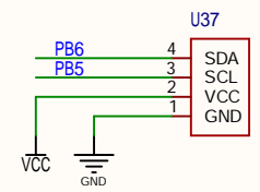
OLED显示屏
