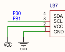
OLED显示屏
