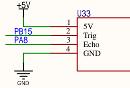
超声波模块
