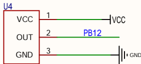
DHT11温湿度
