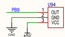
光电红外
