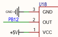
DHT11温湿度传感器
