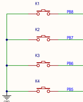
按键
