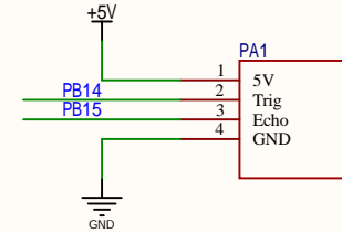
超声波传感器
