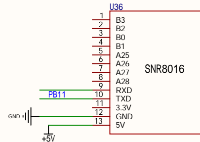
语音识别模块
