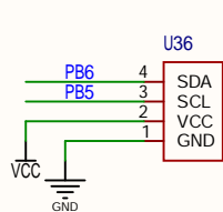
OLED屏幕
