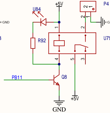
加湿器
