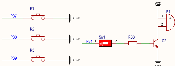
蜂鸣器
