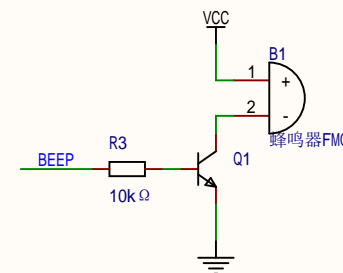
蜂鸣器
