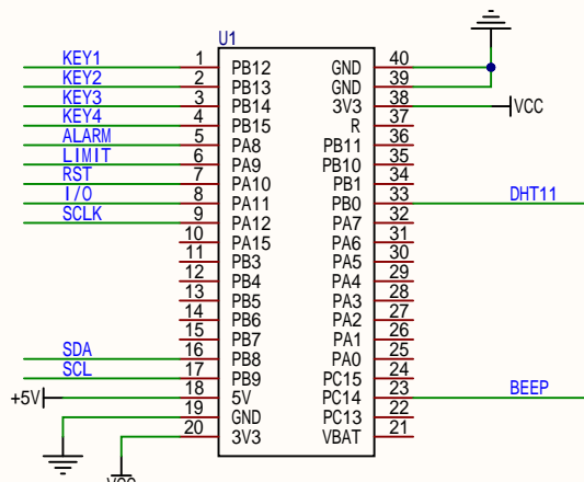
STM32F103C8T6单片机
