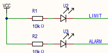
指示灯
