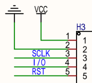
DS1302时钟模块
