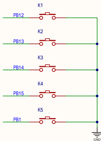
按键
