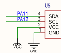
OLED显示屏
