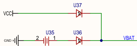
电池
