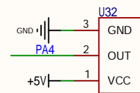
DHT11温湿度
