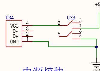
电源模块
