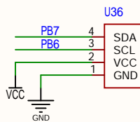
OLED屏幕
