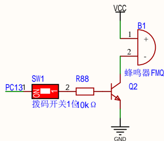
蜂鸣器
