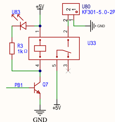
继电器
