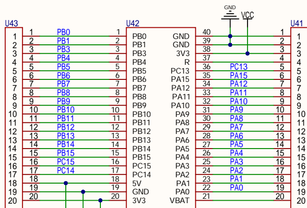
STM32F103C8T6最小系统板
