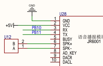
JR6001语音模块
