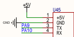
测试接口
