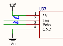
超声波模块
