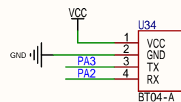
蓝牙模块
