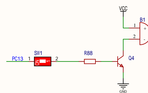
蜂鸣器
