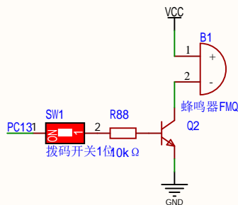
蜂鸣器
