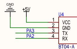
BT04-A蓝牙
