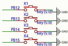
按键
