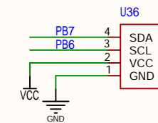
OLED屏幕
