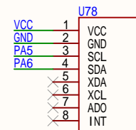
MPU6050陀螺仪
