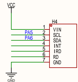
MAX30102心率血氧传感器
