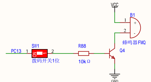
蜂鸣器
