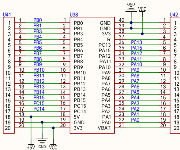
STM32F103C8T6系统板
