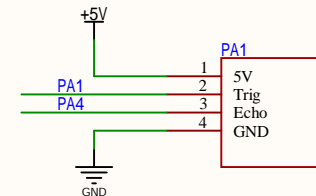
超声波传感器
