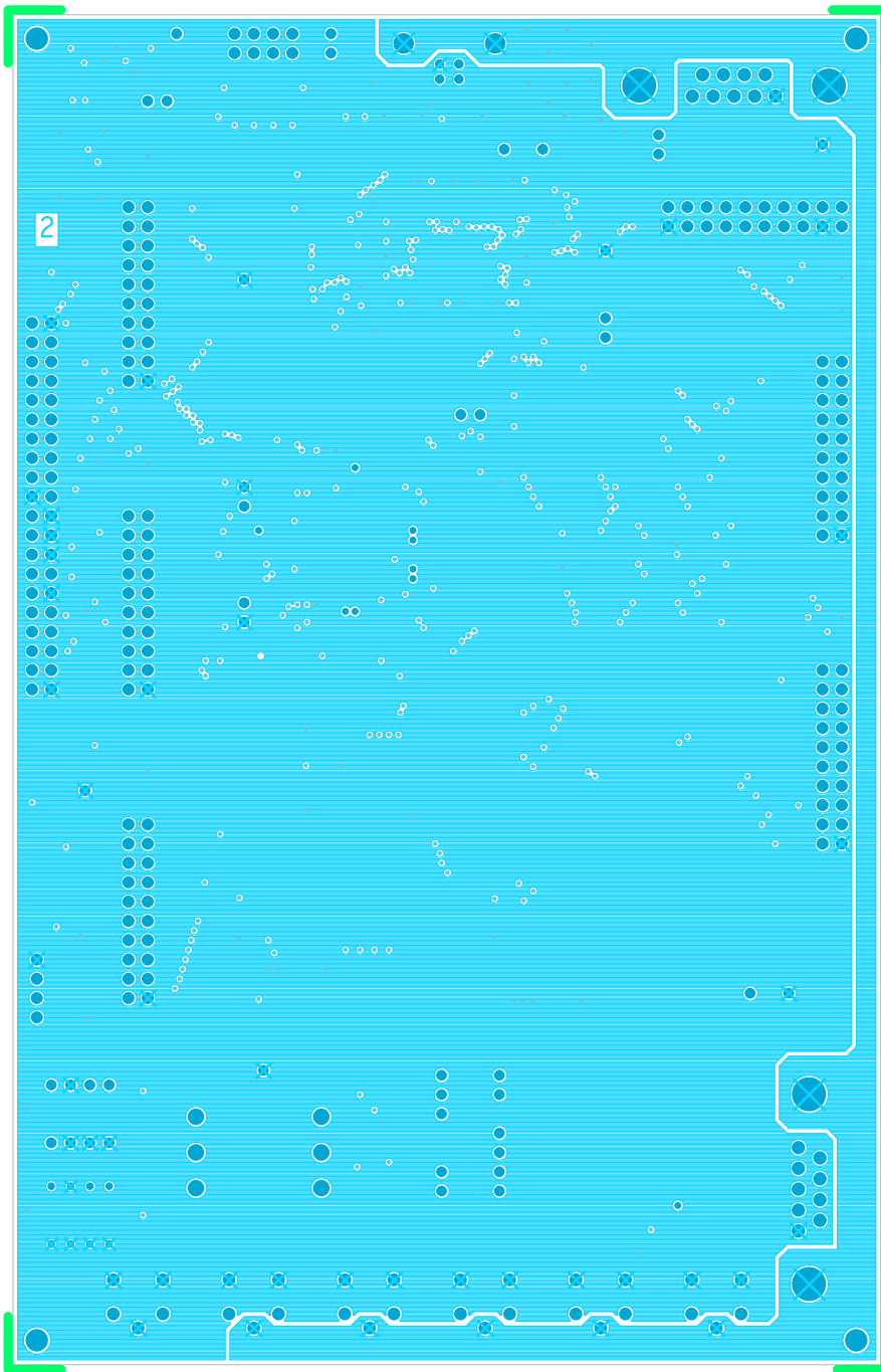
PDC-9086 REV*A LAYER 2 GND
