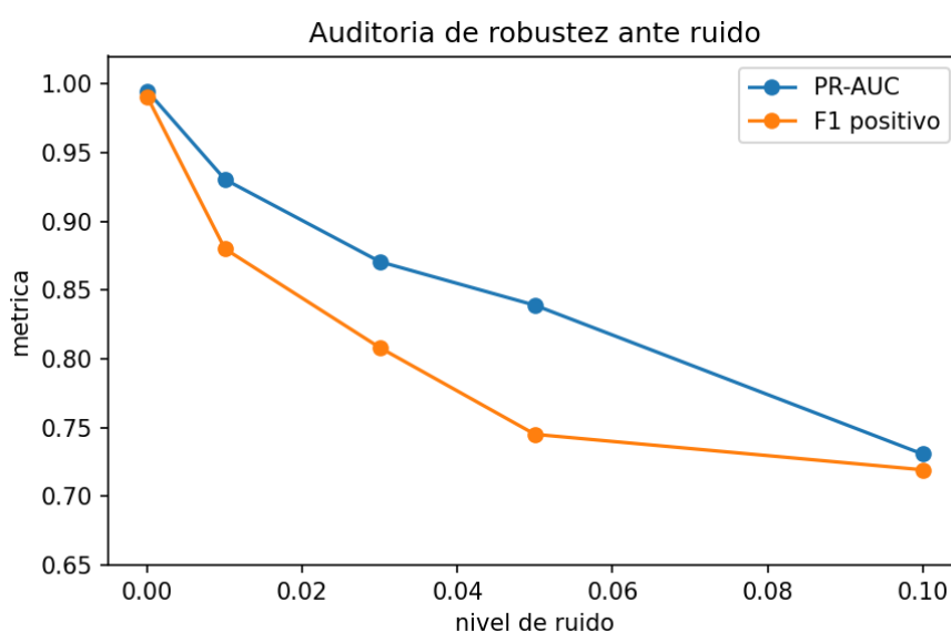
Figura 10: Auditoría de sensibilidad ante ruido en variables numéricas
