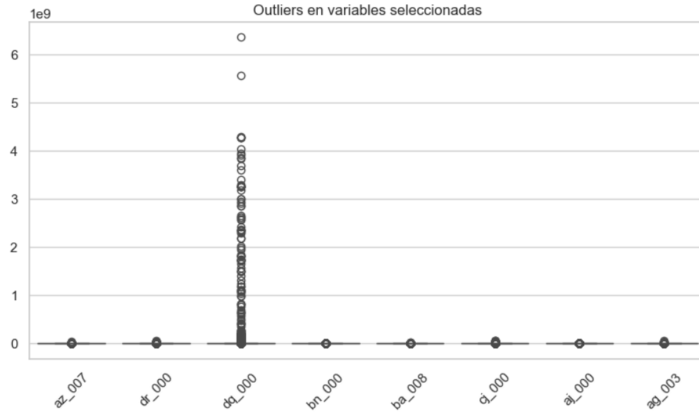
Figura 4: Boxplots de variables seleccionadas para revisar escalas y valores extremos
