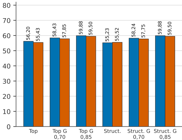
LoRA v2
