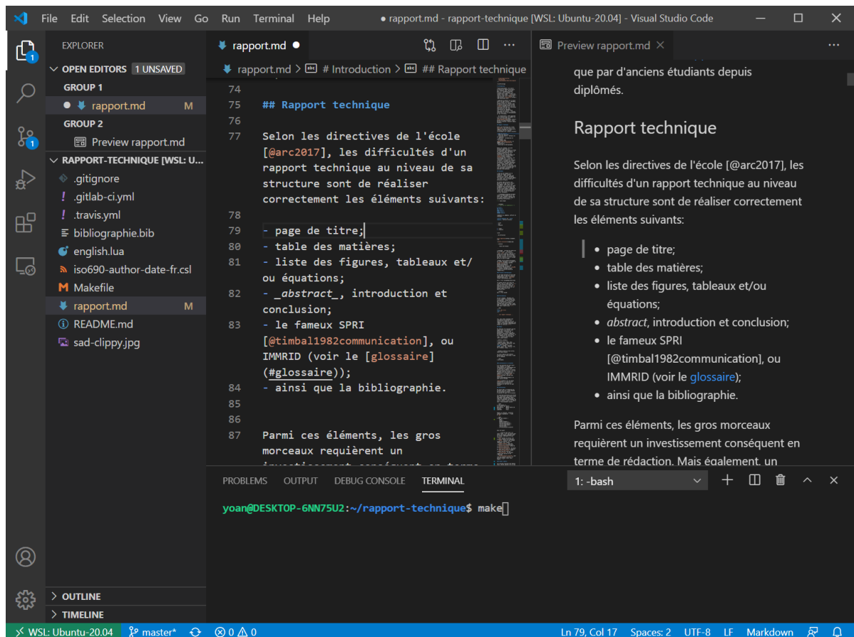
Figure 1.1: Édition avec VS Code
