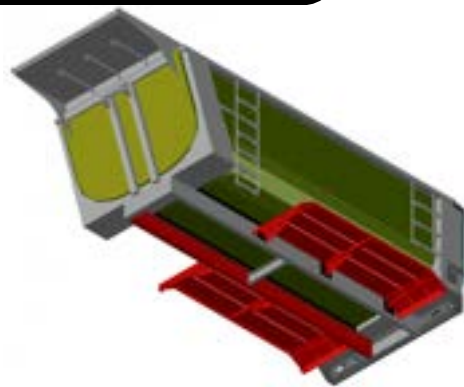
LEVANTAMIENTO PARA FABRICACION DE CAJA DE CAMION
