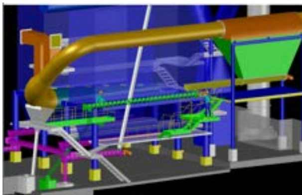
DISEÑO Y PROPUESTAS DE DIRECCION DE DUCTOS, VALVULAS ROTATORIAS, TOLVAS, MEZZANINNES, ESCALERAS
