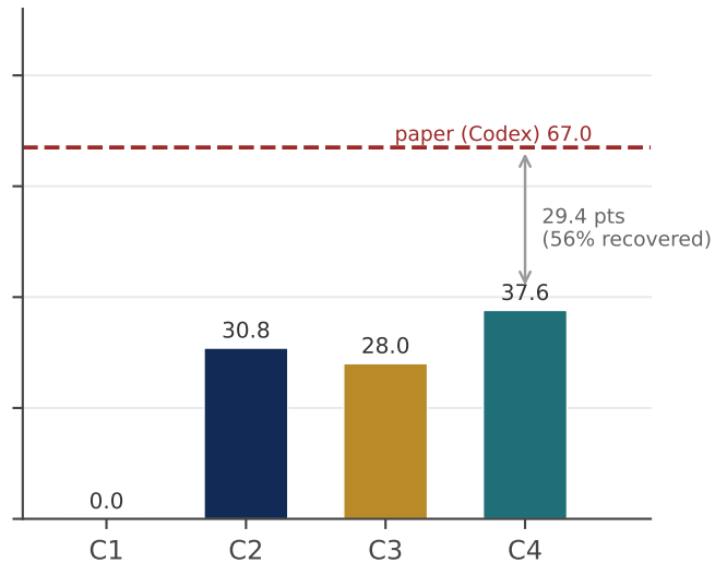
RefCOCO+ / testA
