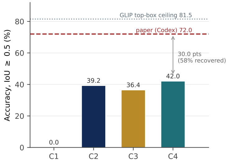
RefCOCO / testA
